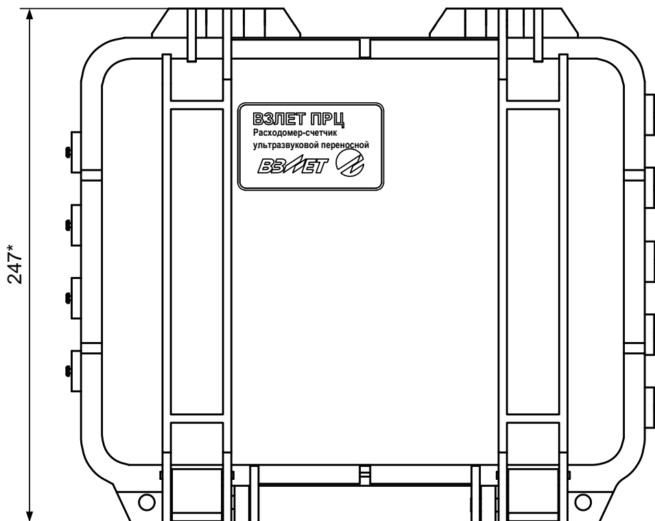
а) вид со стороны крышки
