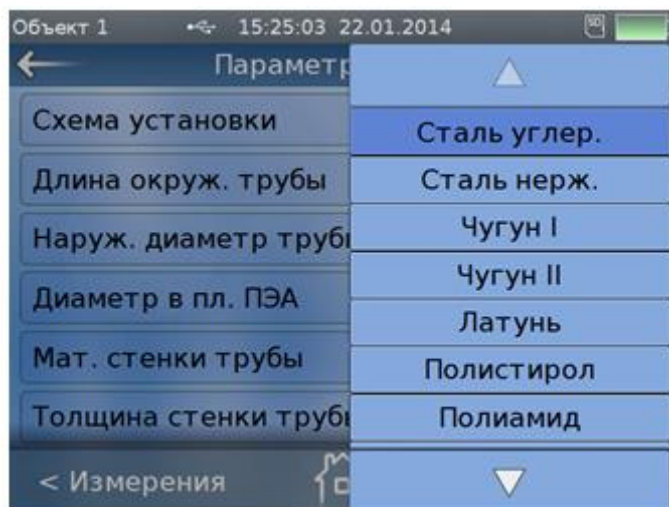
Рис.7. Пример индикации выбора списочных параметров в окне «Мат. стенки трубы» меню «Параметры трубы».
