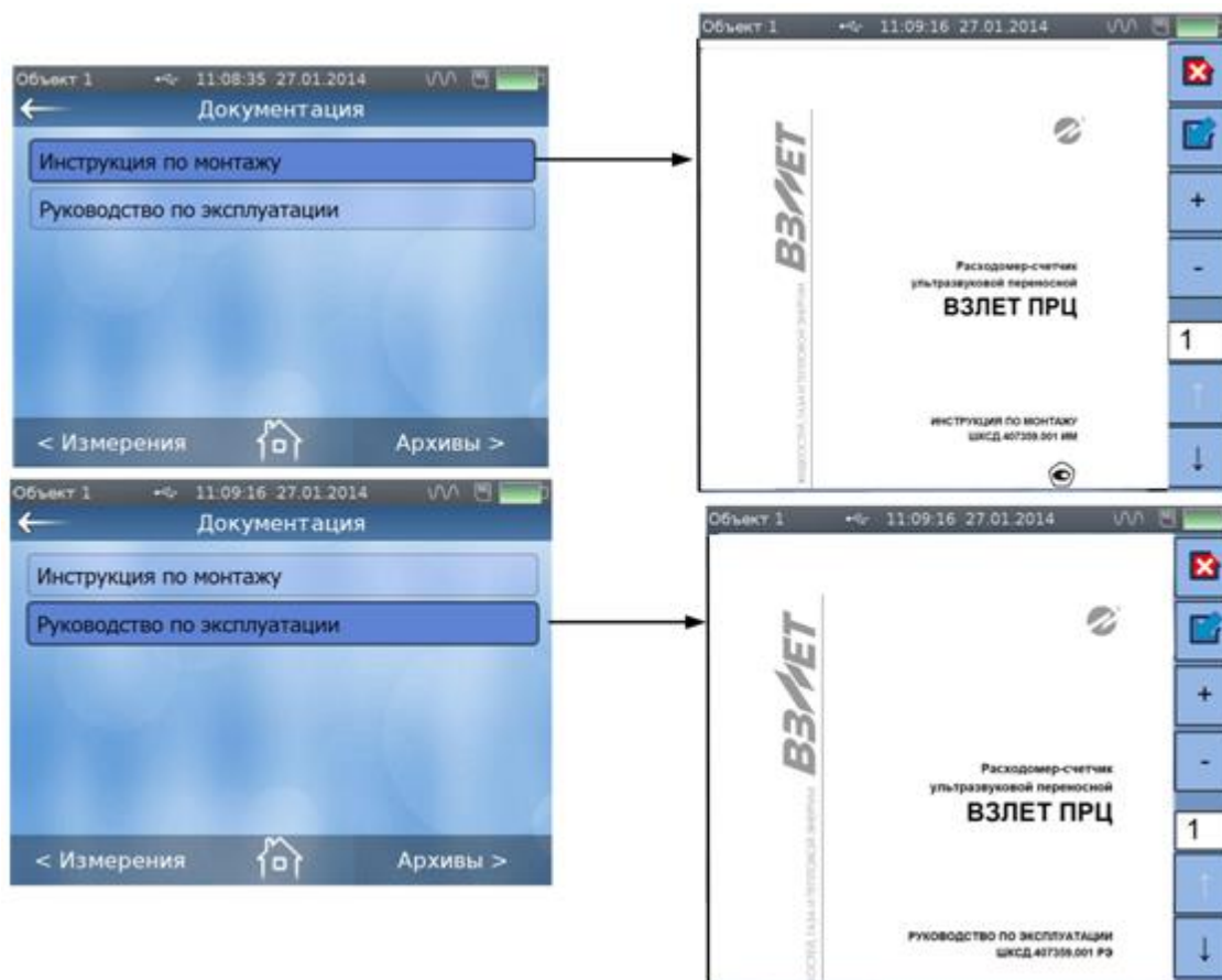
Рис.18. Окно «Документация».
