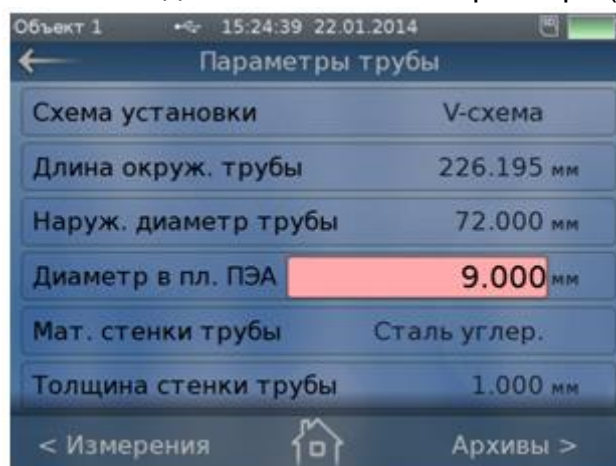
Рис.6. Ошибочно введенное цифровое значение параметра «Диаметр в пл. ПЭА».
