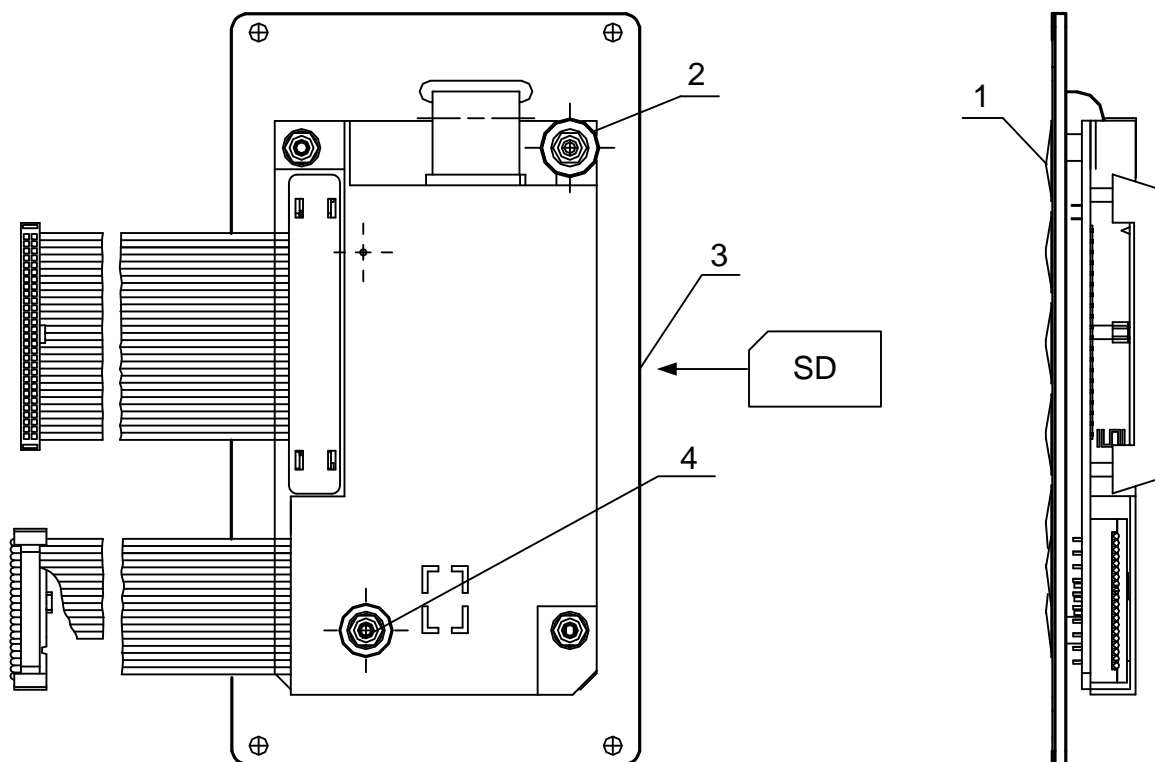
1 – клавиатура; 2 – пломбировочная чашка; 3 – паз для установки карты памяти; 4 – углубление в экране для пломбирования.
