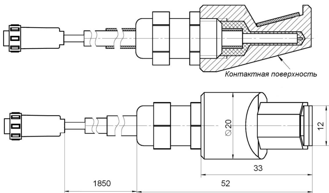
Рис.А.6. Термопреобразователь ТПС-Н.
